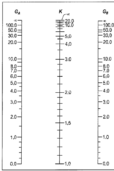
Şekil 6.2 – Yanal yerdeğiştirme önlenmemiş sistemlerde burkulma boyu katsayısı, K
